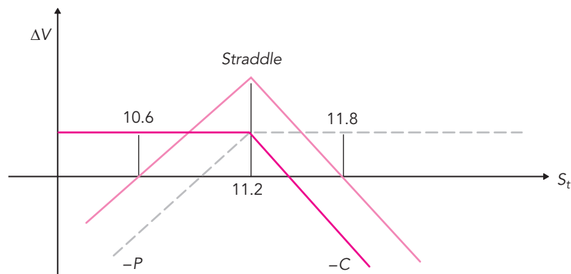
Figura 13.13 Straddle corto.
